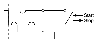
Presse jack 6,3mm per avviamento con fader ④
