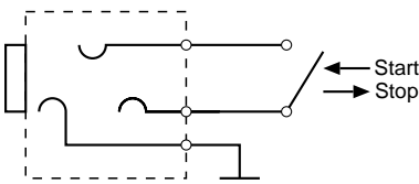
toma jack 6,3 mm para el arranque eléctrico ④
